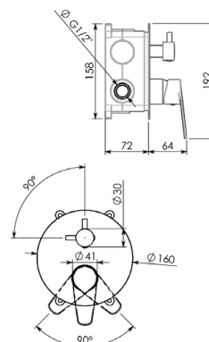
MXCO05 Bateria natryskowa podtynkowa z przełącznikiem z boksem montażowym
