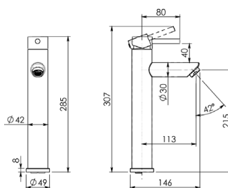
MXGA02 Bateria umywalkowa
