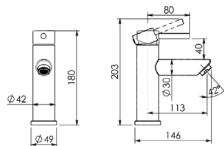
MXGA01 Bateria umywalkowa
