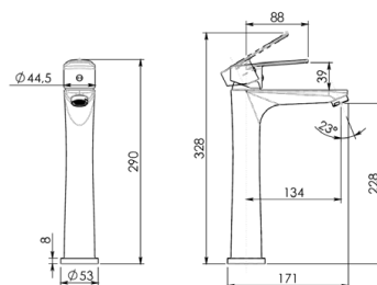
MXCO02 Bateria umywalkowa
