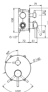
MXGA05 Bateria natryskowa podtynkowa z przełącznikiem z boksem montażowym
