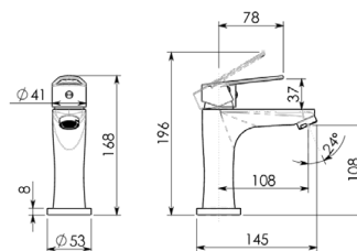
MXCO01 Bateria umywalkowa
